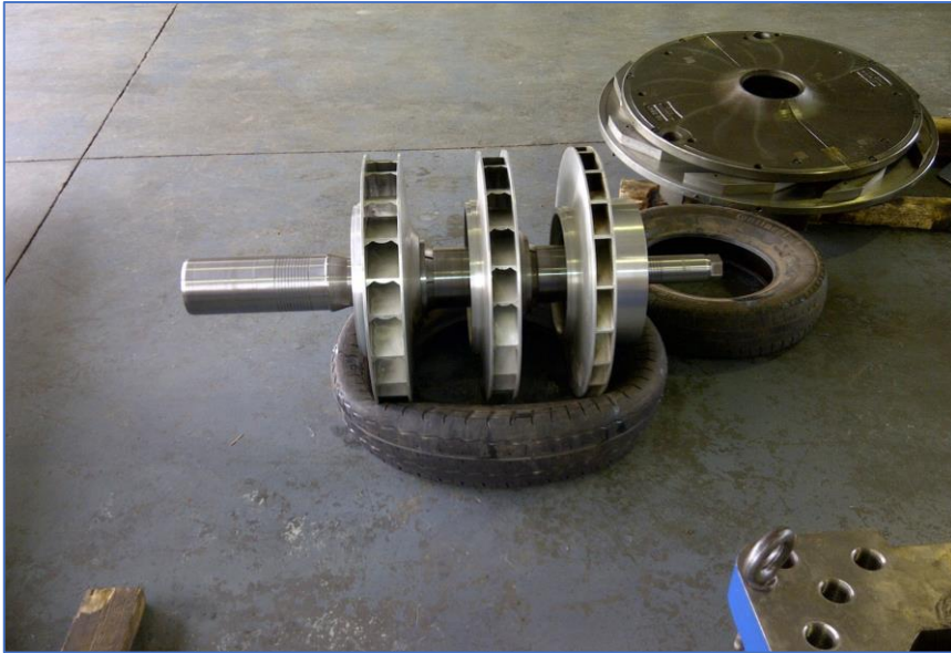
York OM 338 A Compressor disassembly
